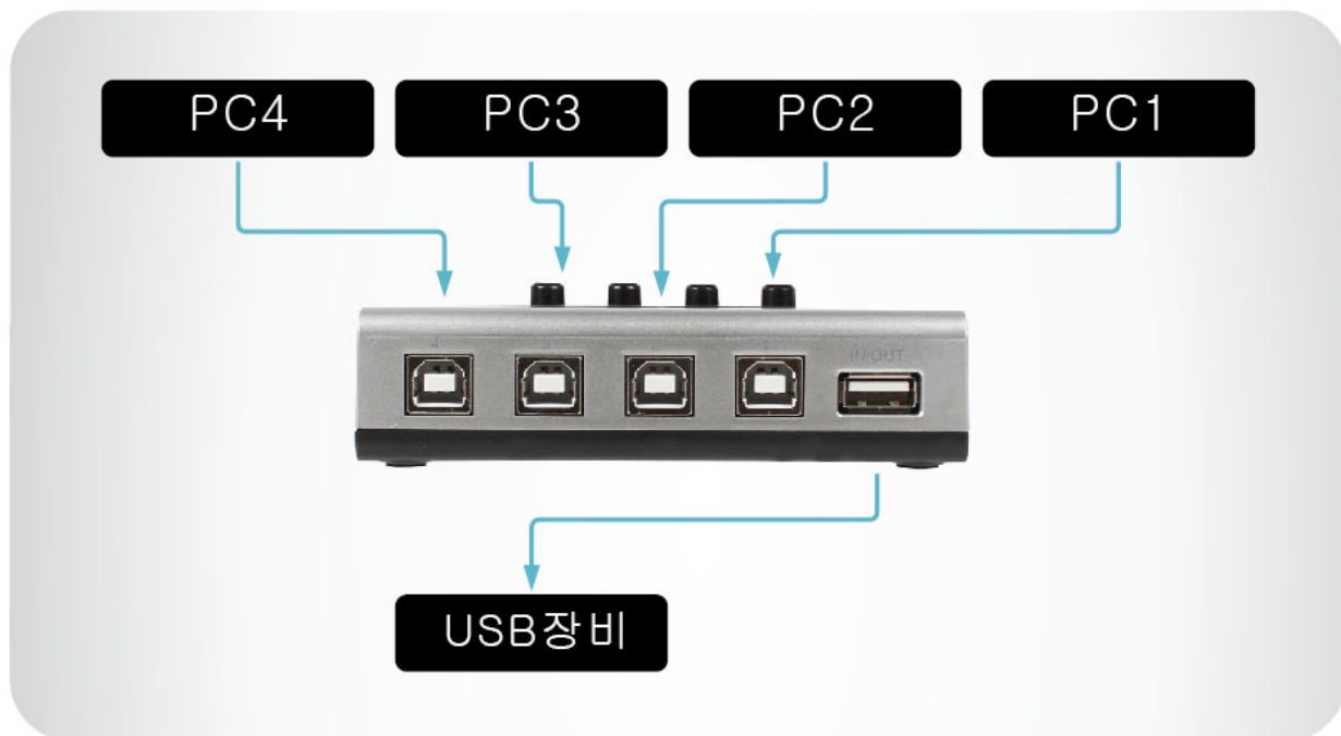
<NM-US14 제품 연결도>
